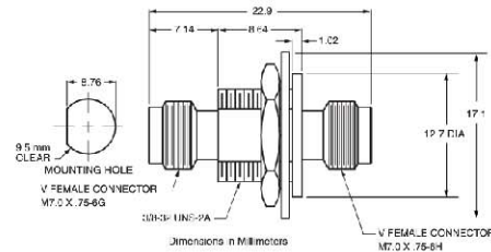
V232 outline
