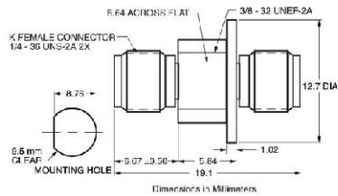
K232B outline
