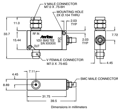
V251 outline
