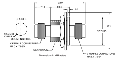
V232 outline
